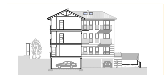
SECCION
